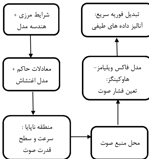
شکل ۴- فلوچارت شبیه سازی [۲۳]
