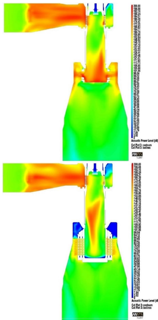
شکل ۱۰- کانتور سطح فشار نویز در صفحه X=0 mm:
